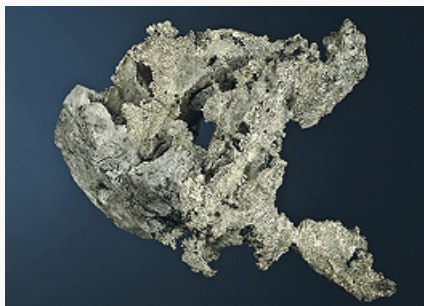
Серебро самородное.
