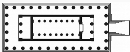
Храм Зевса в Олимпии. План.
