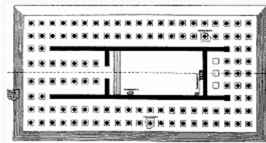
Диптер (план).
